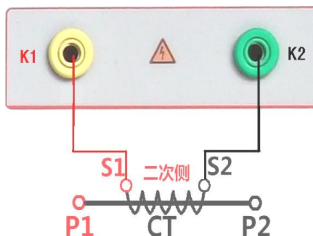
图 5，CT 励磁特性接线图
